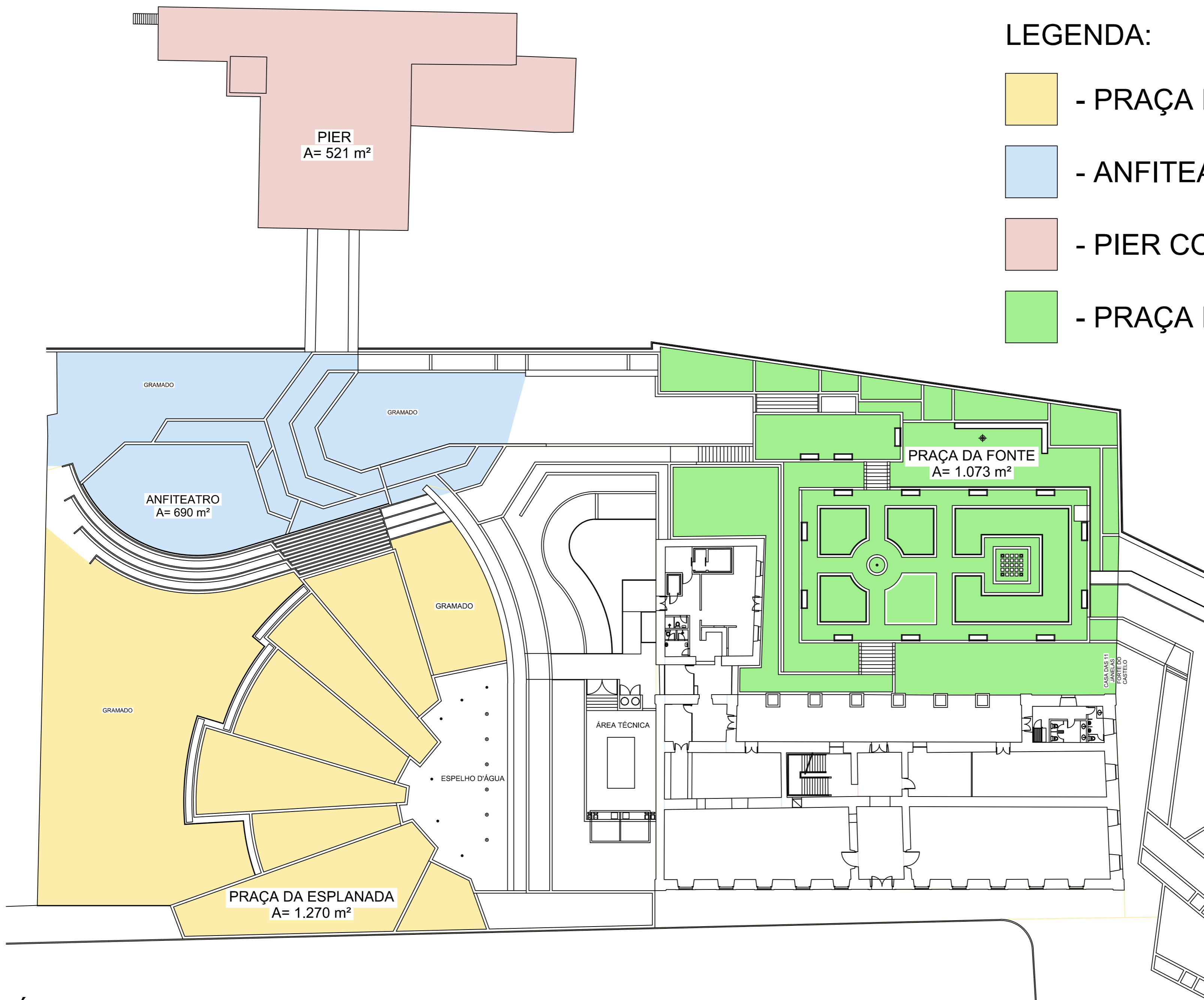
ÁREA EXTERNA - CASA DAS 11 JANELAS S/ESCALA
