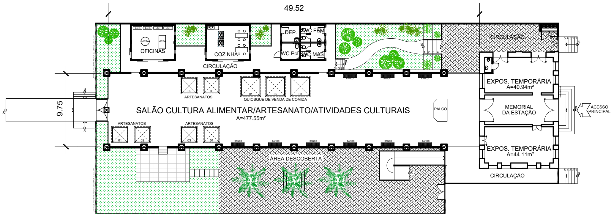
PLANTA BAIXA - ESTAÇÃO FERROVIÁRIA DE ICOARACI SEM ESCALA
